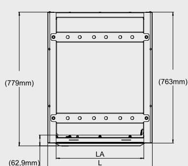
VISTA SUPERIOR
